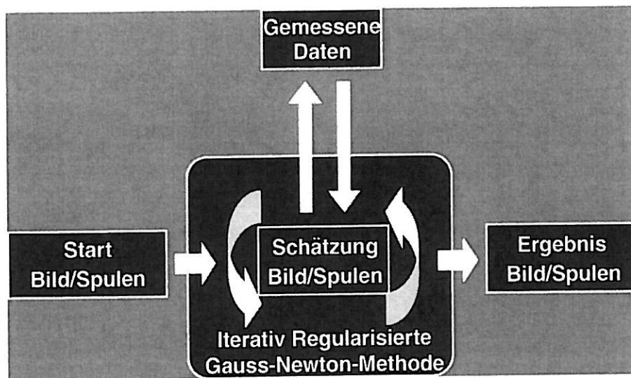
Abbildung 2: Das Prinzip der iterativen Bild-Rekonstruktionen durch regularisierte nicht-lineare Inversion. Bei dieser Berechnung werden ein MRT-Bild und die Intensitätsprofile der eingesetzten Empfangsspulen geschätzt und die dazu gehörenden Daten berechnet. Anschließend wird das Schätzbild durch iterativen Abgleich der synthetischen mit den gemessenen Daten gezielt verändert und in mehreren Schritten optimiert. Dieser Prozess kann erheblich verbessert werden, wenn sich die Lösungsvielfalt durch eine Regularisierung des Iterationsprozesses mit Zusatzkenntnissen über das gewünschte Bild und die Spulenprofile einschränken lässt.
